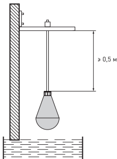
Рис. 2 – Монтаж RL-1
