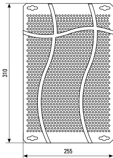
Рис. 2б – Монтажная плата большая
