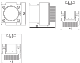
Рис. 1 - Приставка выдержки времени ПВЭ
