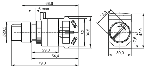
Переключатель D8-11X2; переключатель D8-11X22; переключатель D8-20X3; переключатель D8-20X33
