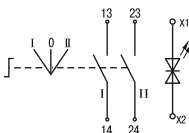
Переключатель D8-20XD3
