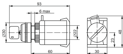
Переключатель AKS-22
