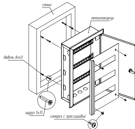
Рис. 1. Схема монтажа
