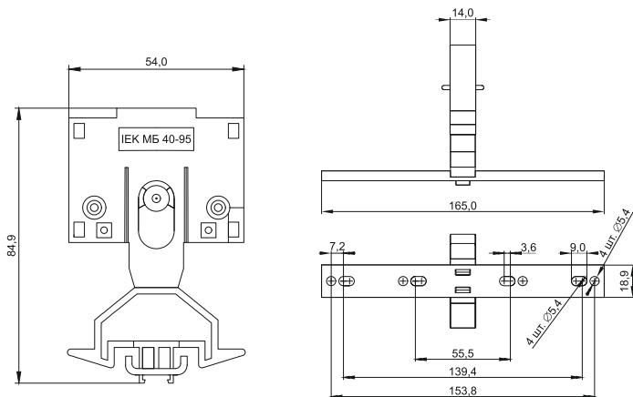
б) Механизм блокировки для КМИ (40А-95А) / b) Locking mechanism for KMI (40A-95A)
