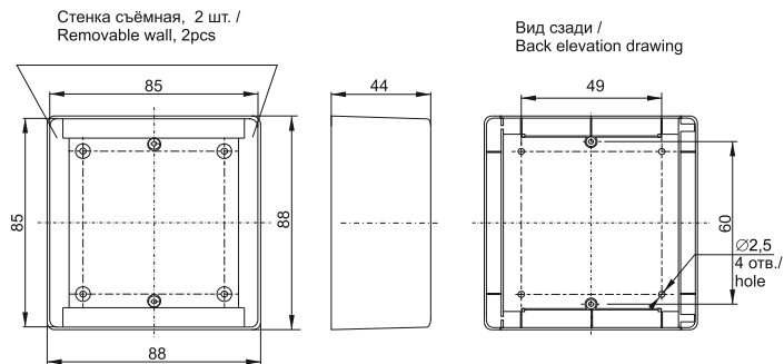
Рисунок 2 – КМКУ артикулы CKK10D-U-1-KXX и EL-KK10D-U-K02 / Figure 2 – KMKU of CKK10D-U-1-KXX and EL-KK10D-U-K02 order codes
