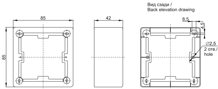
Рисунок 1 – КМКУ артикул CKK10D-U-2-KXX / Figure 1 – KMKU of CKK10D-U-2-KXX order code
