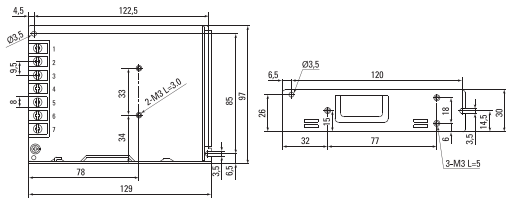
Рис 3. Габаритные размеры (MPS-100W-24)
