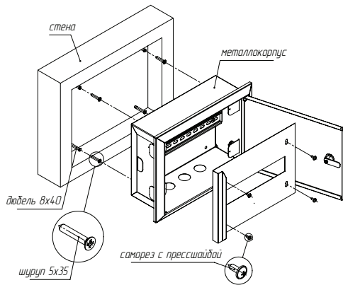
Рис. 1. Схема монтажа
